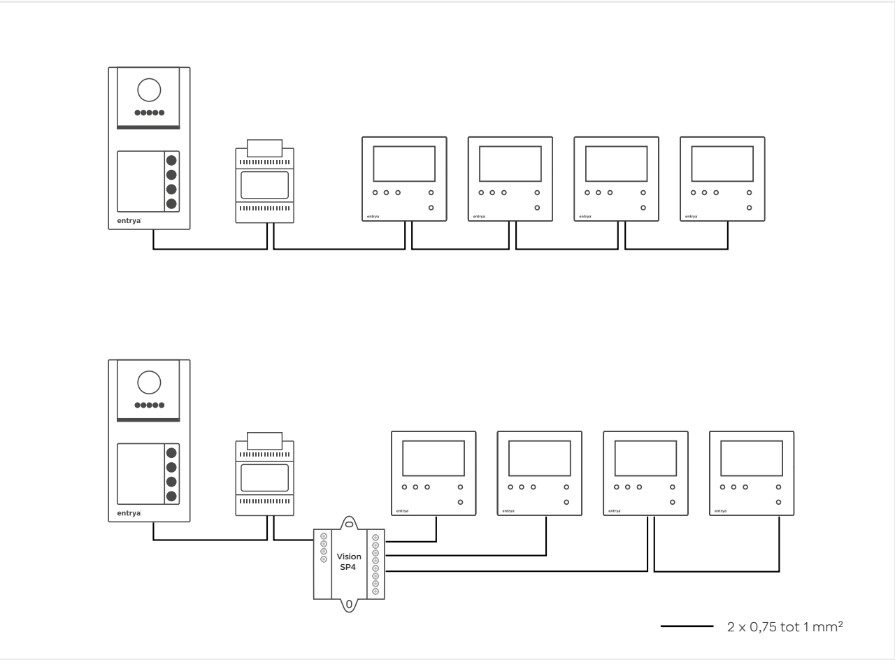
Schema voor een klein appartementsgebouw
