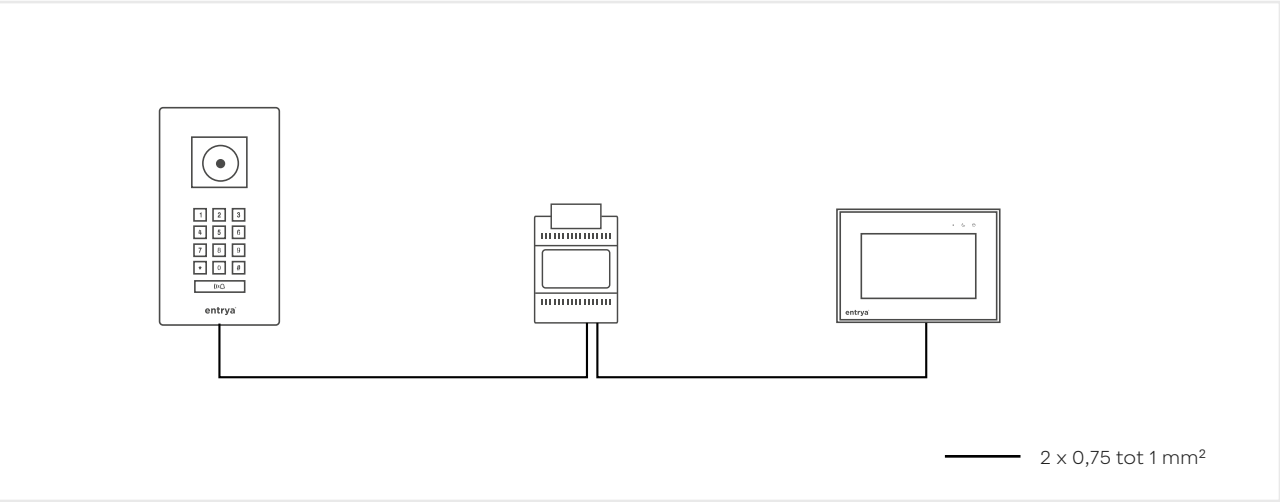
Schema voor residentiële woningen
