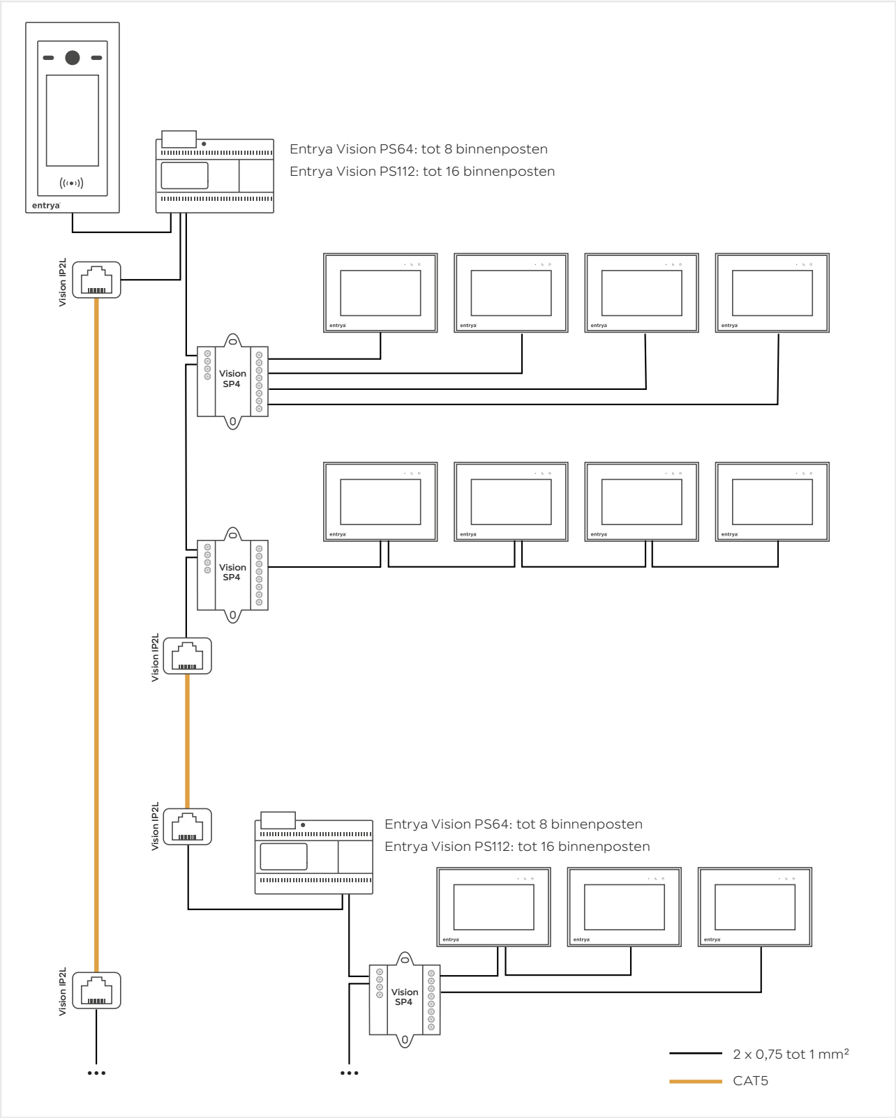
Schema voor een groot appartementsgebouw
