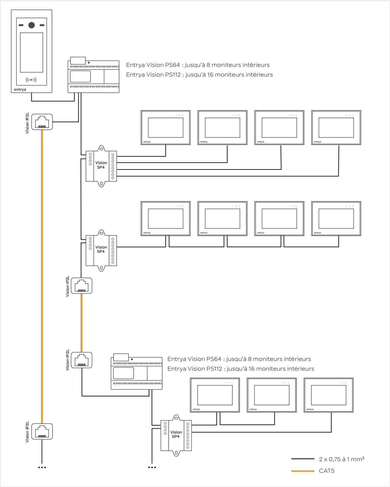
Schéma pour grand immeuble à appartements
