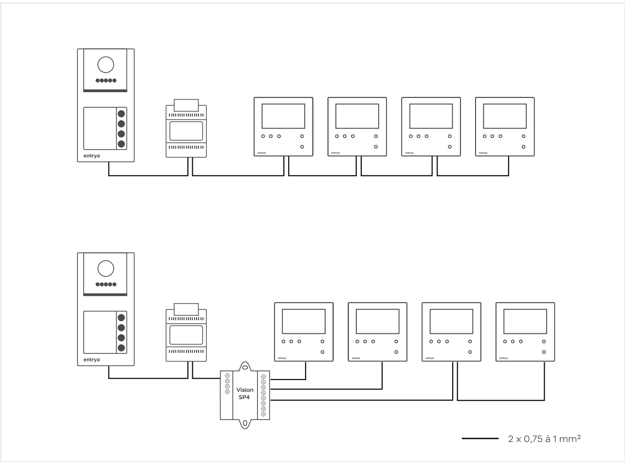
Schéma pour petit immeuble à appartements
