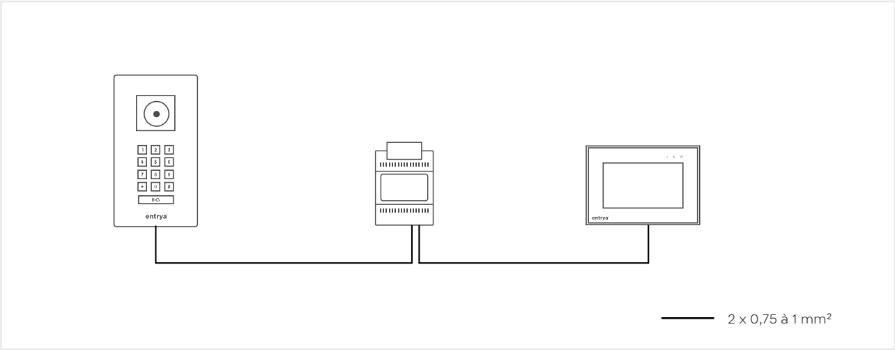
Schéma pour maisons individuelles
